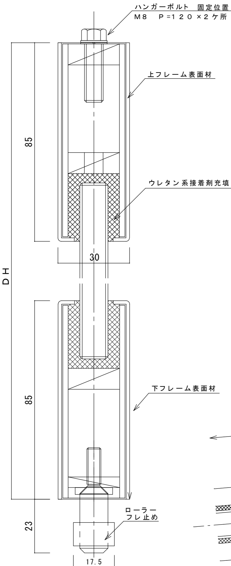
A-A断面図 S=1/1
