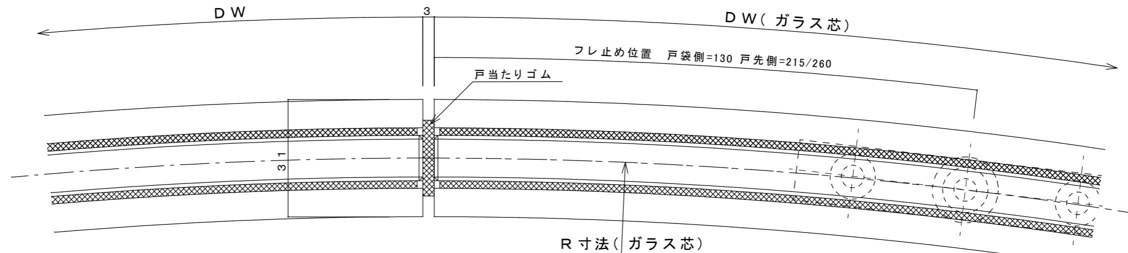
B-B断面図 S=1/1
